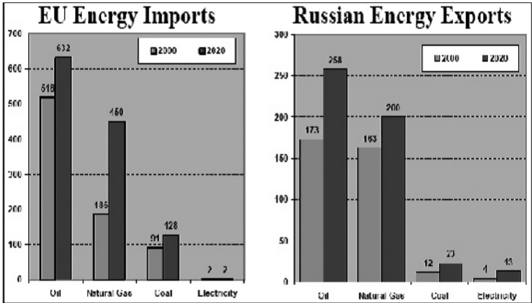
Fig. 3 – Importazioni ed esportazioni di energia equivalente a milioni di tonnellate di petrolio Fonte: Commissione europea, Tendenze al 2030. Federazione Russa – La strategia della Russia fino al 2020
