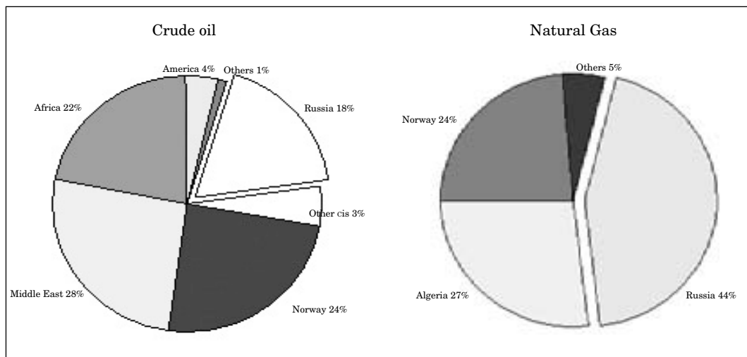
Fig. 2 – I rifornimenti di idrocarburi nell’Ue nel 2001 Fonte: Piper Jeff – Commissione europea, DG Energia e Transporti
