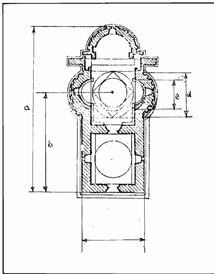
Plan inițial al bisericii Voroneț, fără pridvor.
