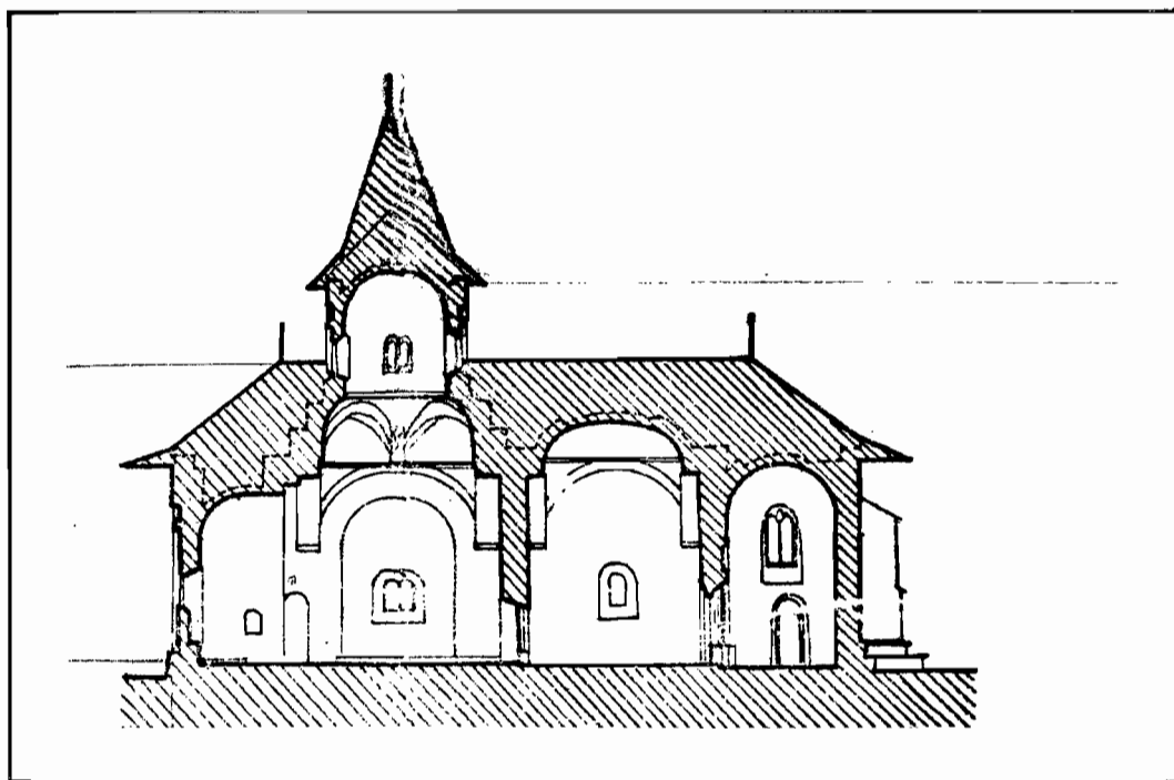
Biserica Voroneț - Secțiune actuală.
